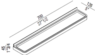
700mm shelf AMEM856
